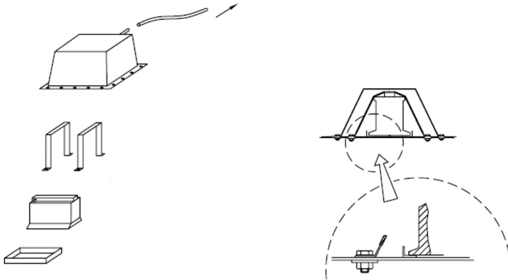
TEKENING 255-10
